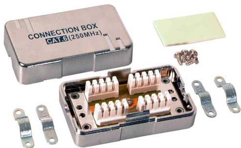
Verbindungsmodul Kat. 6
