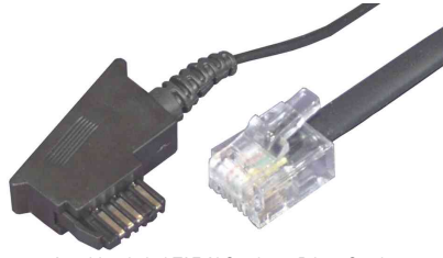
Anschlusskabel TAE-N Stecker - RJ 12 Stecker
